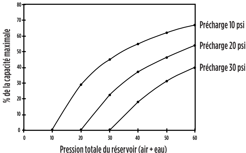
Capacité du réservoir de stockage pressurisé
